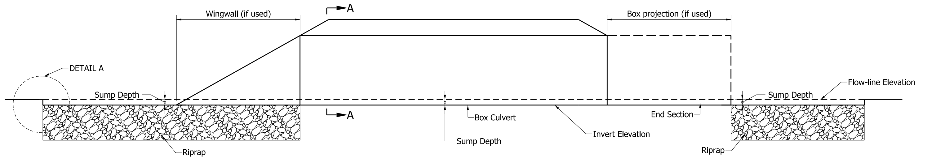
ELEVATION
