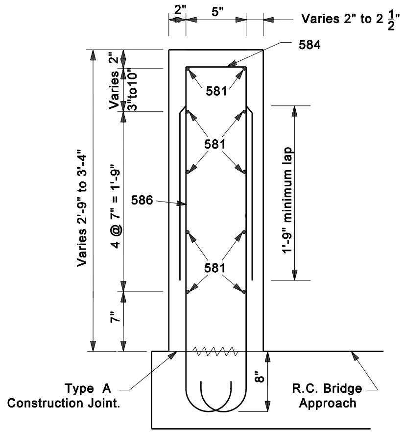
SECTION D-D
