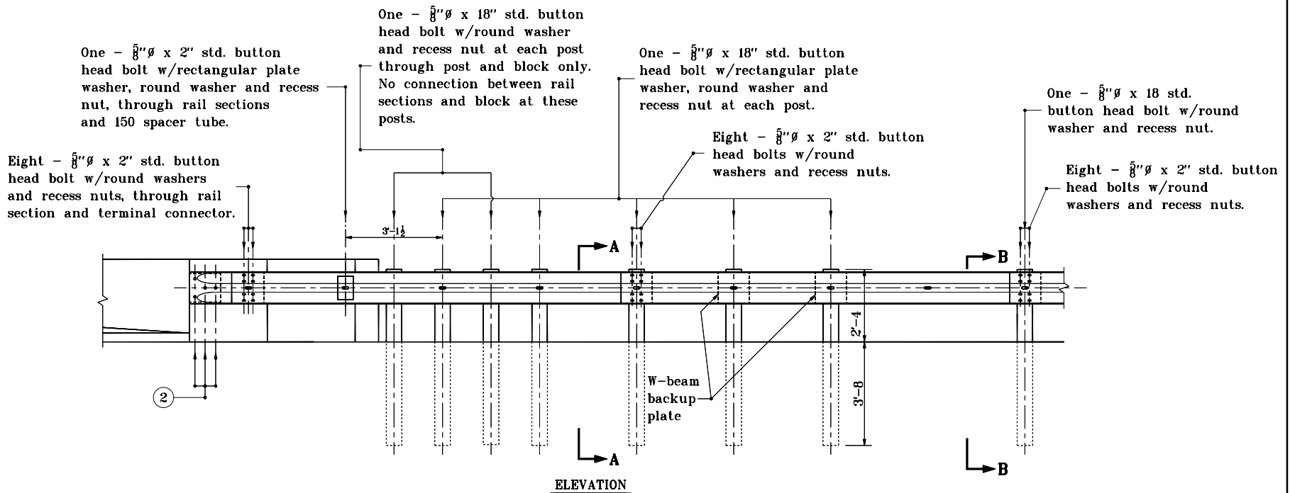
ELEVATION
