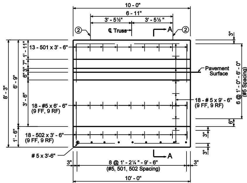
ELEVATION
