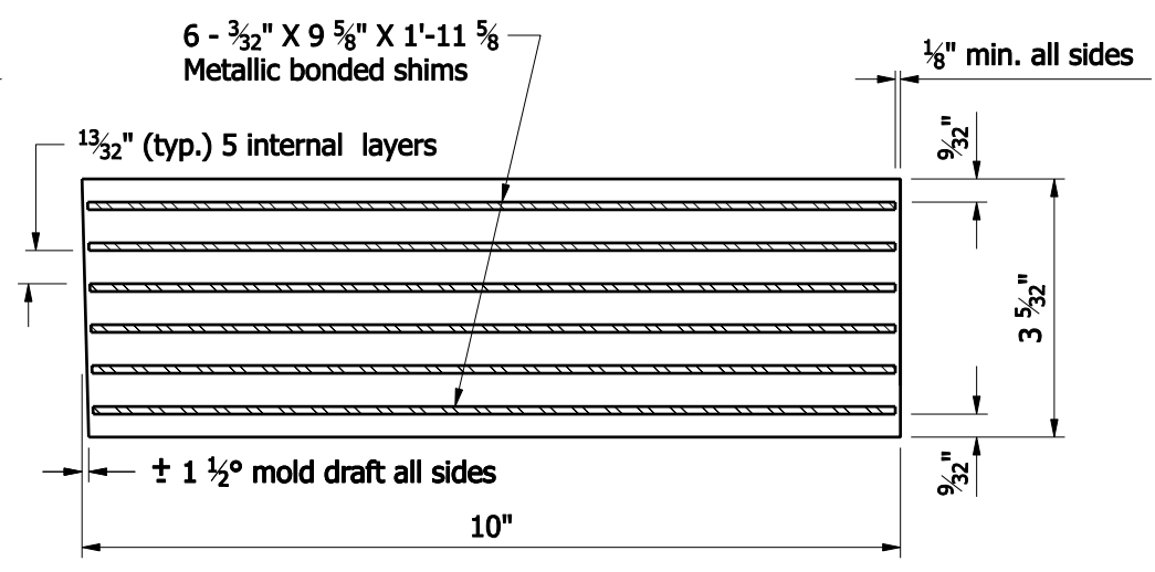
SECTION D-D TYPE 4
