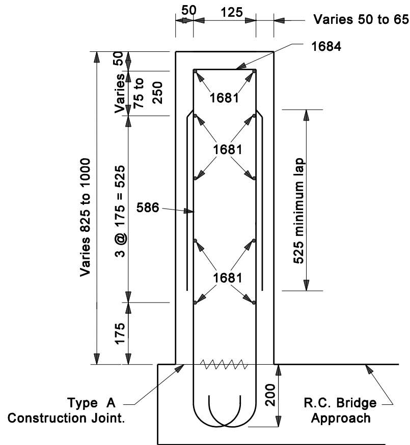
SECTION D-D
