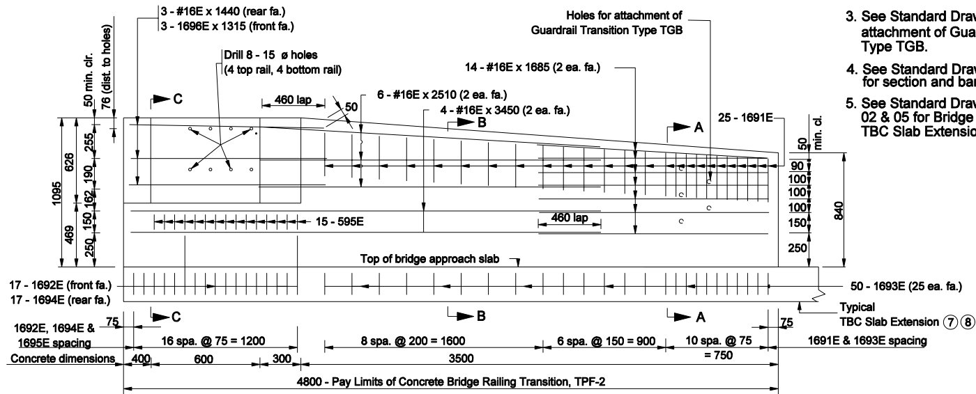
ELEVATION
