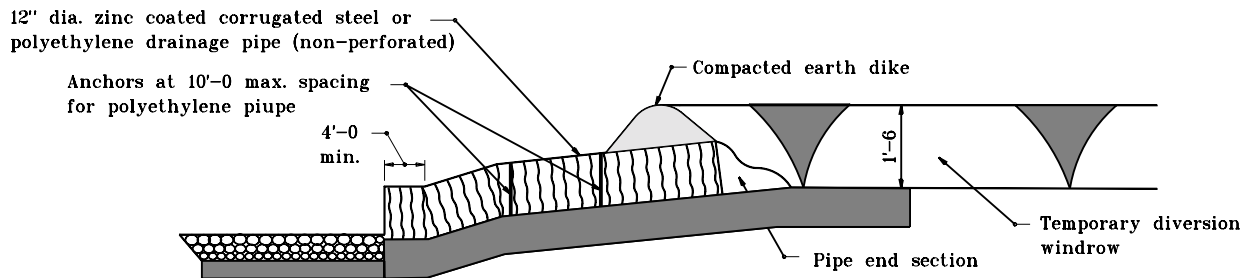
ELEVATION
