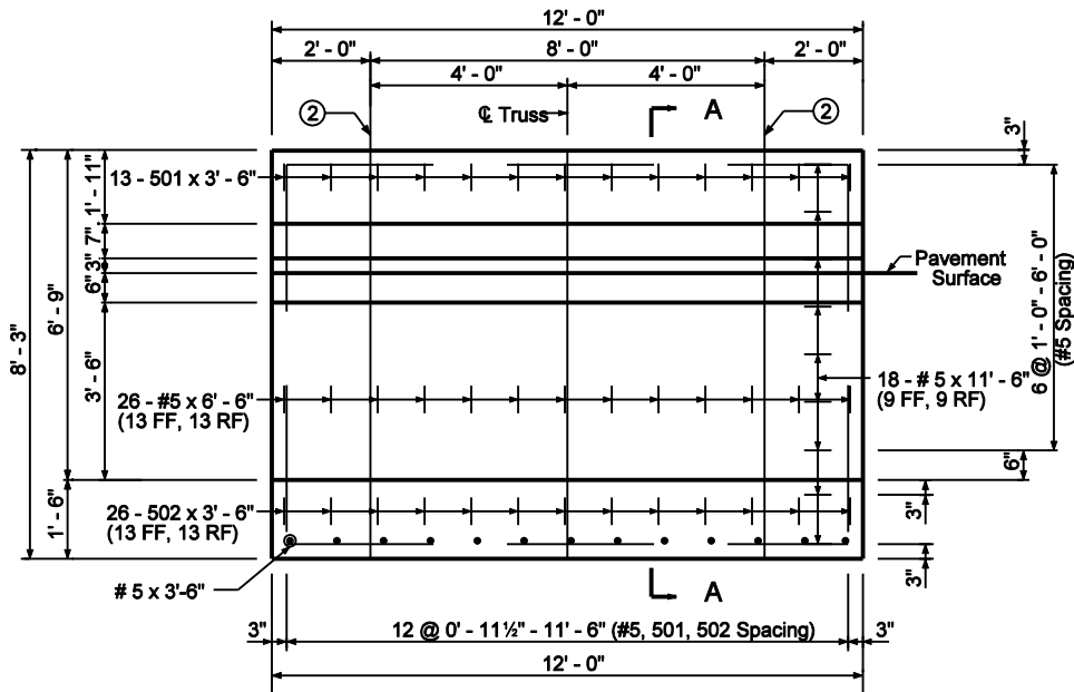
ELEVATION
