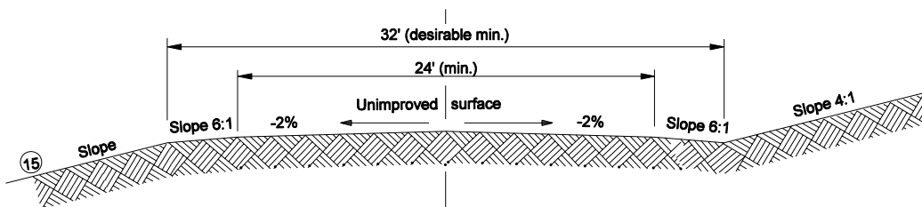
SECTION D-D
