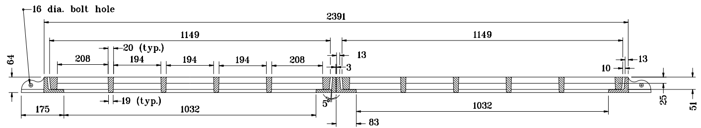
SECTION A-A
