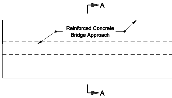
PLAN - END BENT
