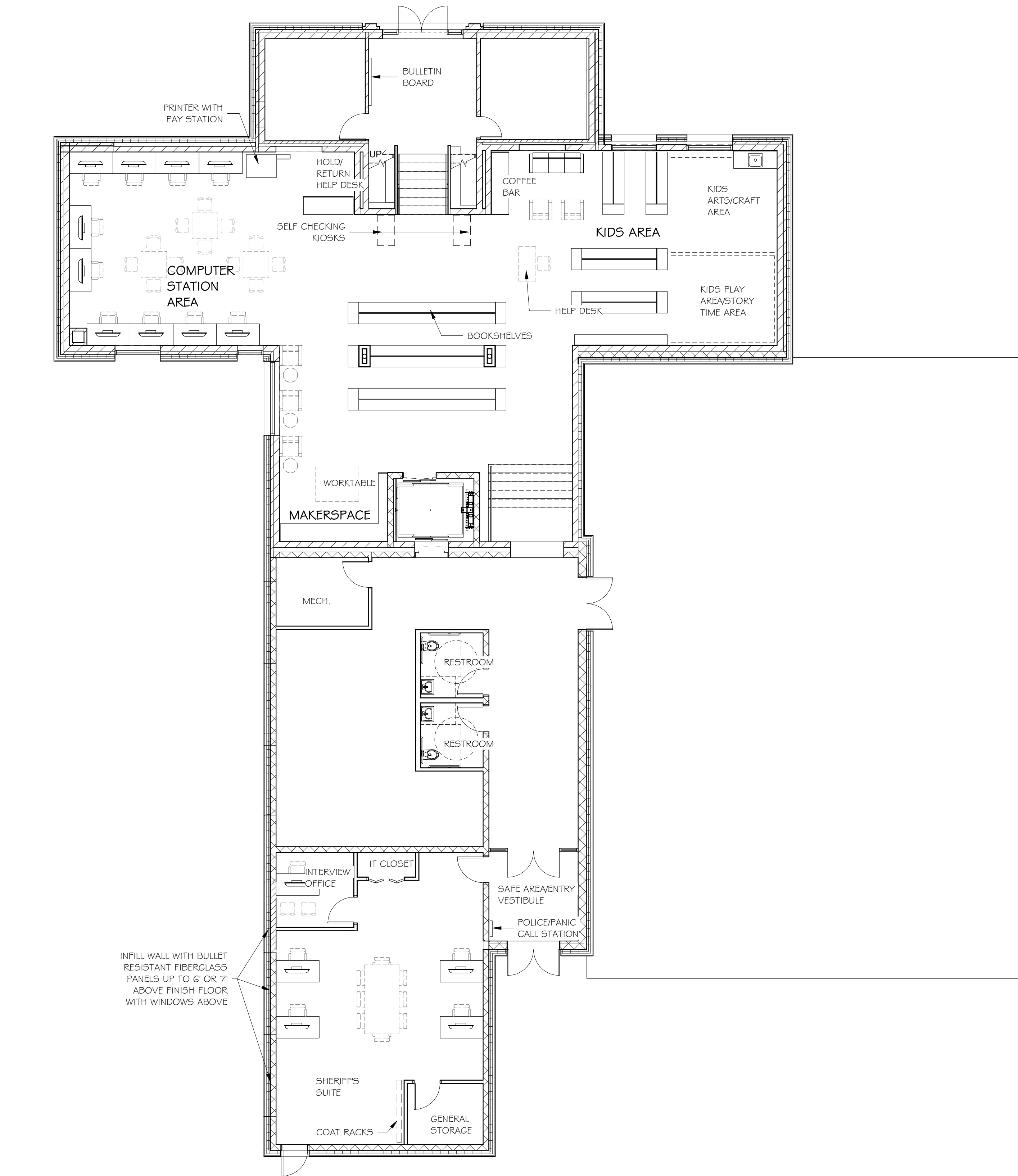
1 LOWER LEVEL SCALE: 1/8" = 1'-0"
